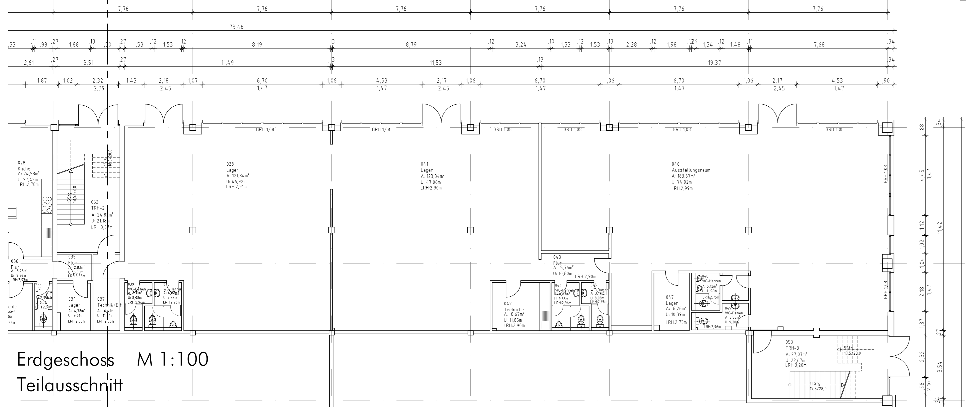
Erdgeschoss M 1:100 Teilausschnitt
