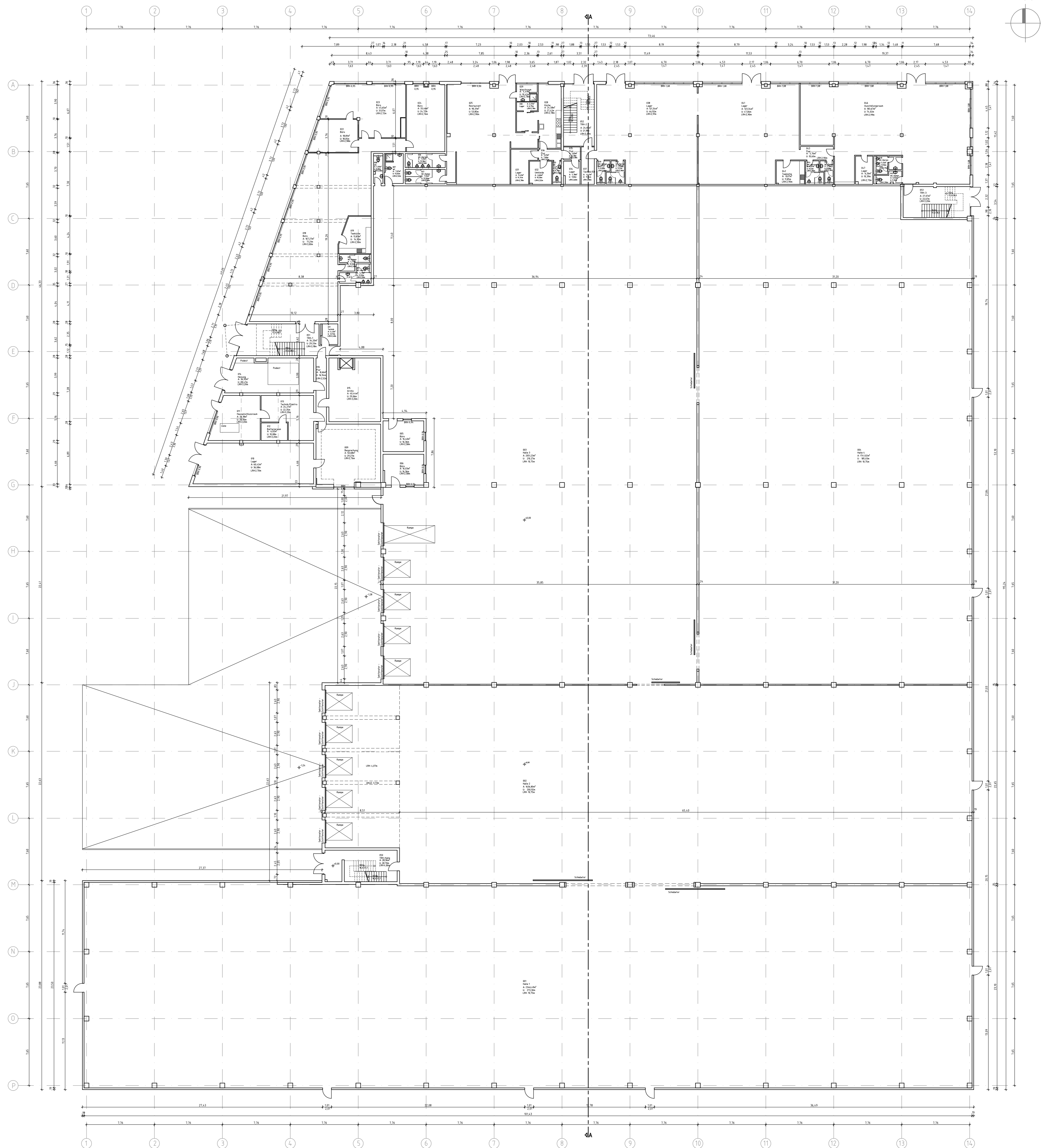
Erdgeschoss M 1:200
