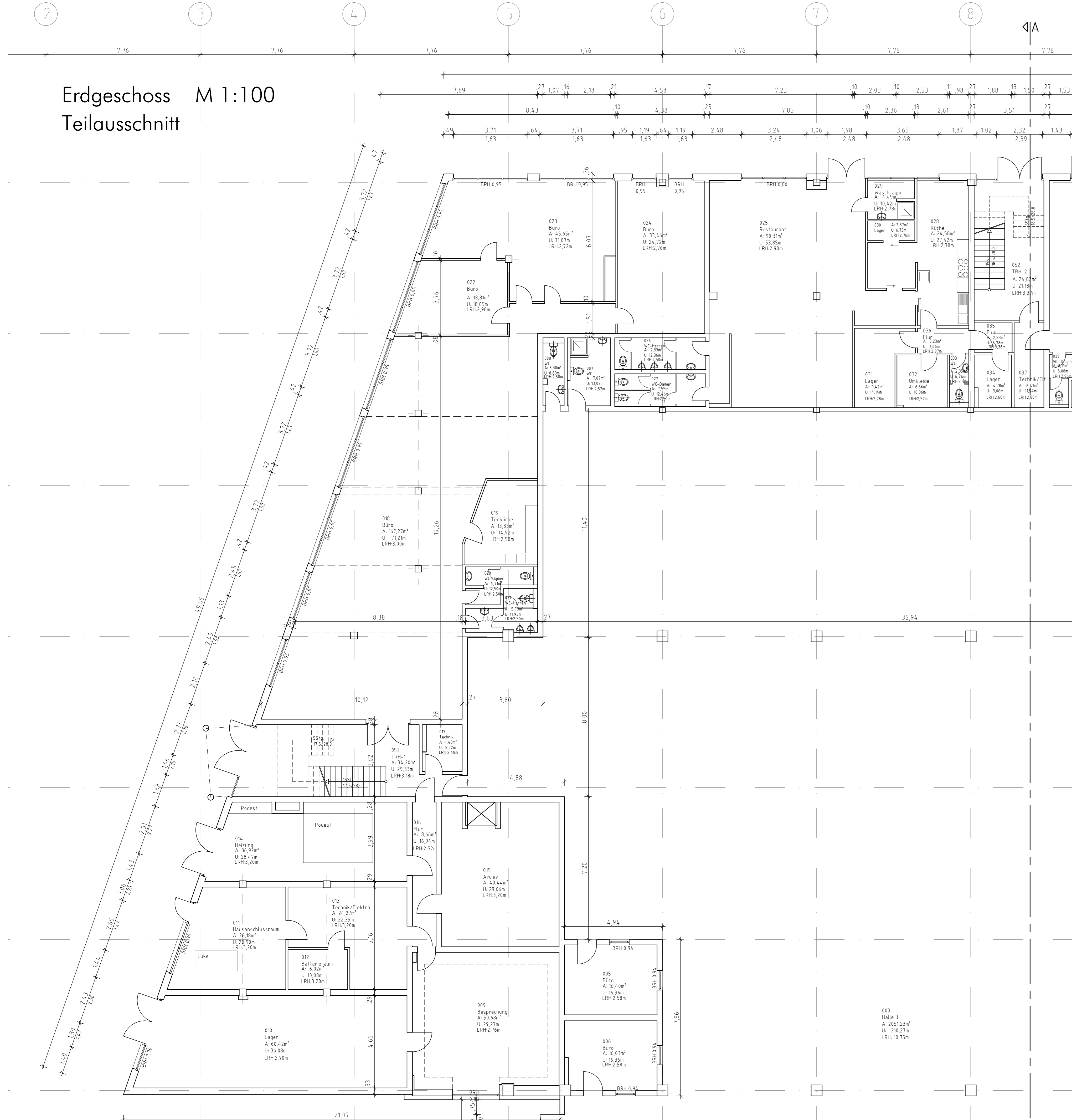
Erdgeschoss M 1:100 Teilausschnitt
